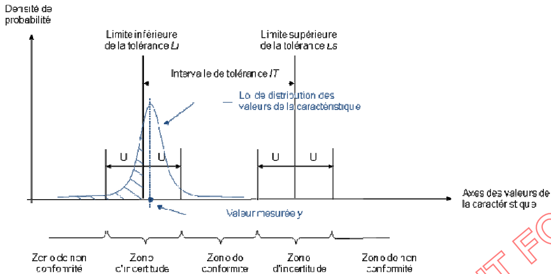
Figure 2 : Probabilité de déclarer conforme un instrument non conforme, approche selon le fascicule FD X07-022
